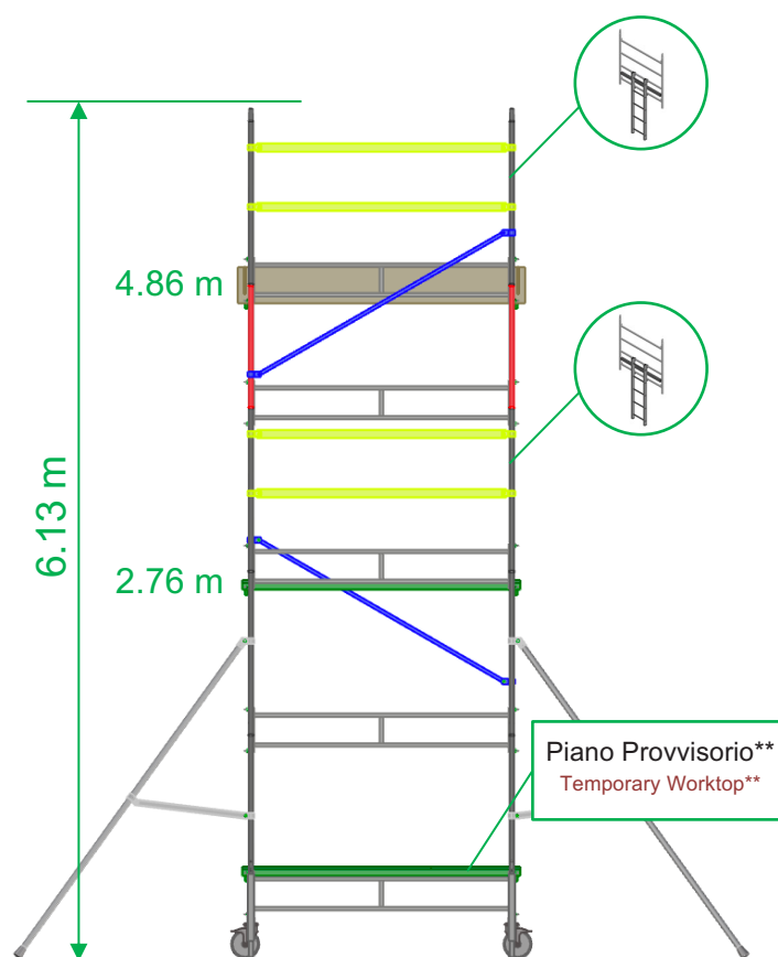
Mod. A+B+C+D4+E : T061SP
