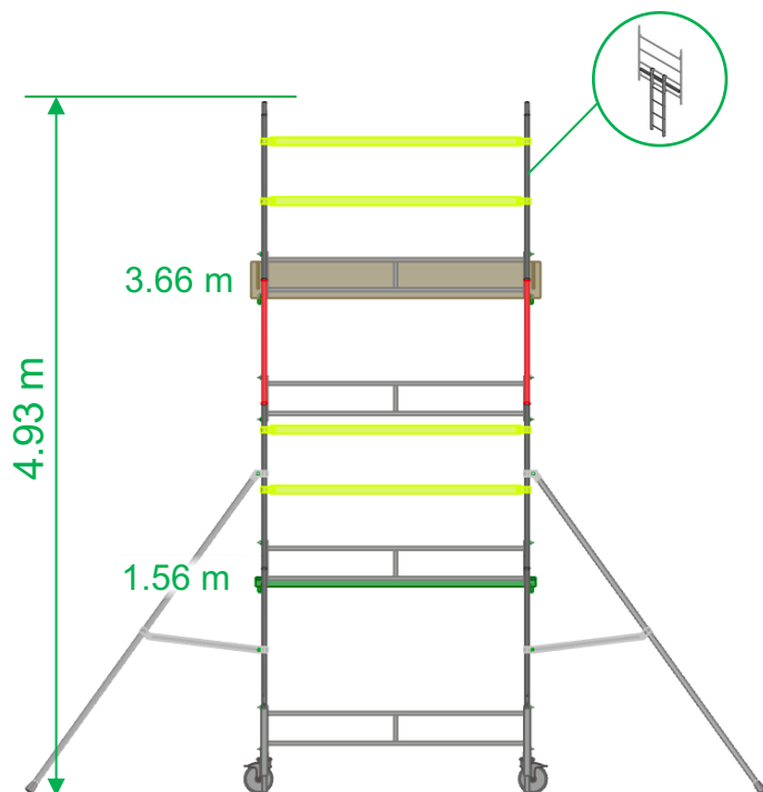
Mod. A+B+C : T049SP
